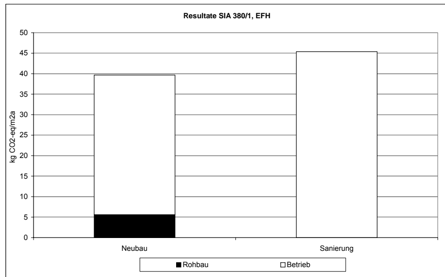
Abbildung 16: Treibhauspotential (in kg CO 2 -eq) für Bau, Betrieb und Rückbau von Einfamilienhäusern nach SIA 380/1 Grenzwert für Neubau bzw. Sanierung. Der Anteil Rohbau (ohne Wärmedämmung) ist separat ausgewiesen.
