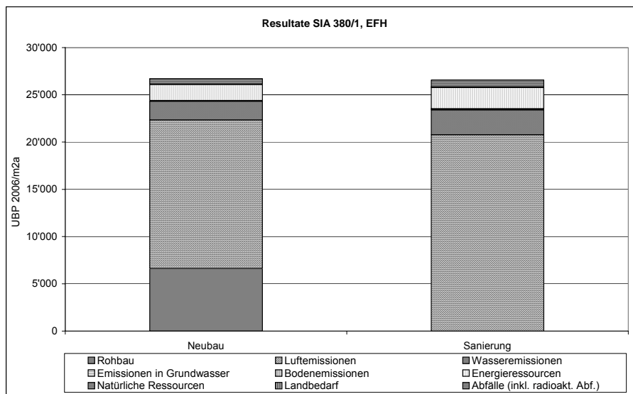
Abbildung 22: Umweltbelastungspunkte 2006/m 2 a (provisorische Ökofaktoren) für Bau, Betrieb und Rückbau von Einfamilienhäusern nach SIA 380/1 Grenzwert für Neubau bzw. Sanierung. Der Anteil Rohbau (ohne Wärmedämmung) ist separat ausgewiesen.
