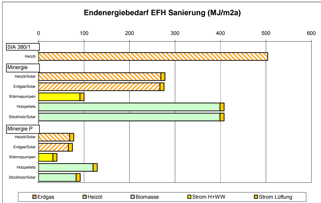
Abbildung 9: Endenergiebedarf EFH Sanierungen
